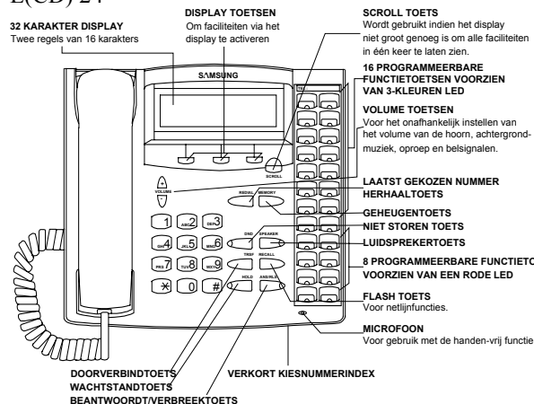
L(CD) 24
